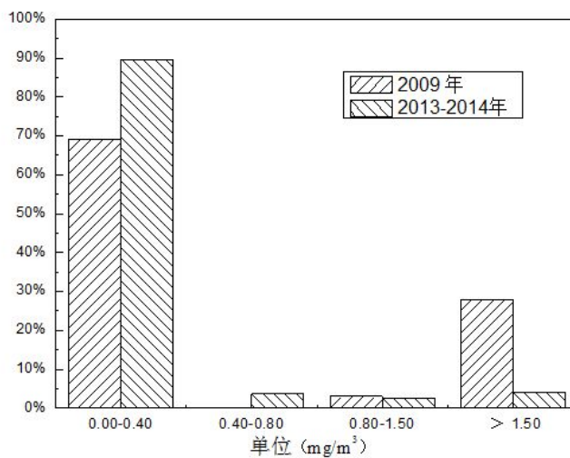
图 7-5 车内空气中乙苯实验结果
